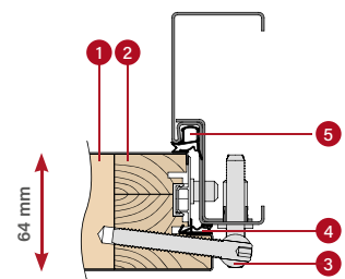
OCEĽOVÁ ZÁRUBŇA
