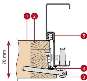
OCEĽOVÁ ZÁRUBŇA
