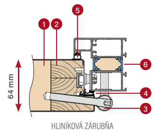
HLINÍKOVÁ ZÁRUBŇA
