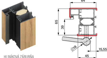
HLINÍKOVÁ ZÁRUBŇA
