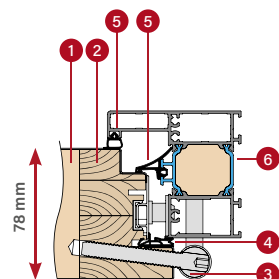
HLINÍKOVÁ ZÁRUBŇA
