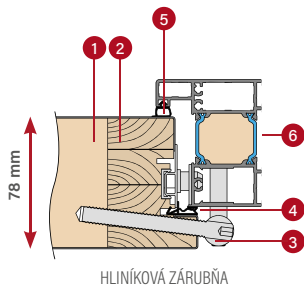
HLINÍKOVÁ ZÁRUBŇA
